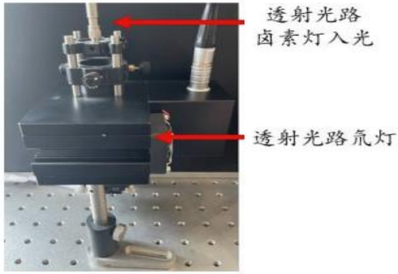
图 18.透射入光光路
