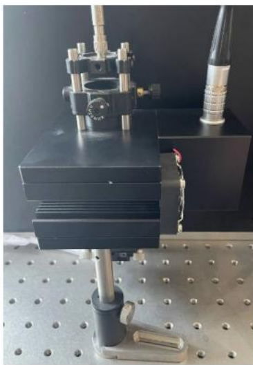
图 19.氙灯-卤素灯光源组合
