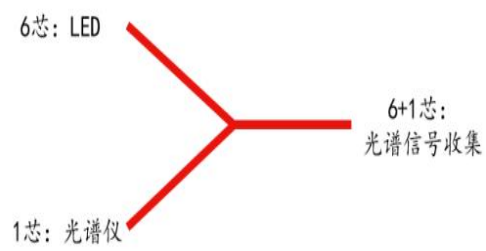
图 16.Y 型光纤图
