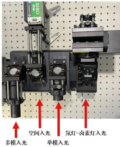
图 13.入光模块组
