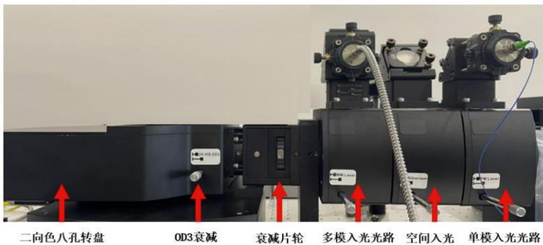
图 10.多路集成反射光路
