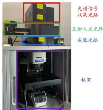
图 6.整体结构图
